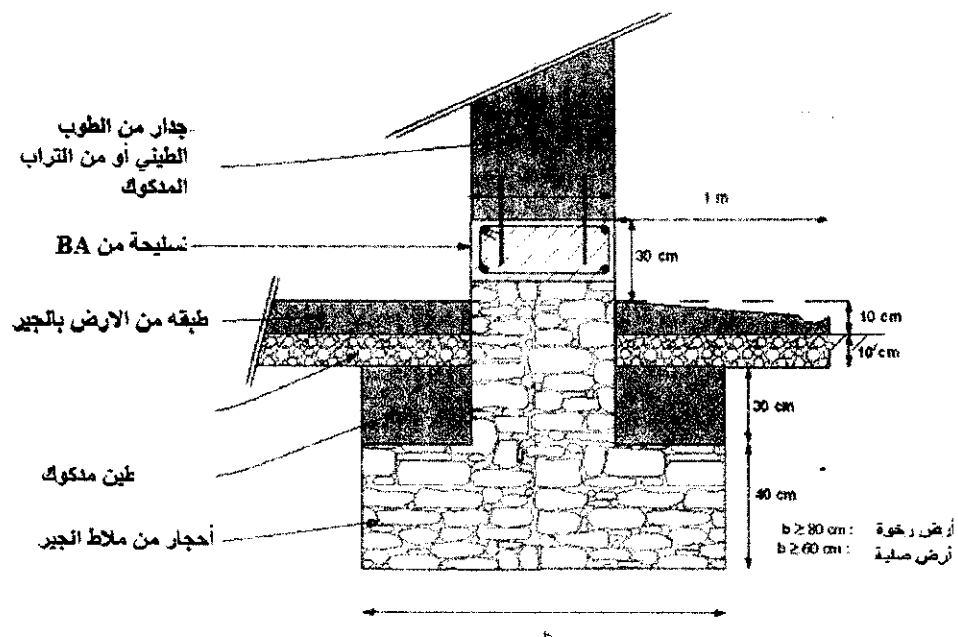
الشكل 48. أساس من البناء الرضعات + مئترات من الخرسانة المسلحة + أعمدة الربط جدار - مئطرة
