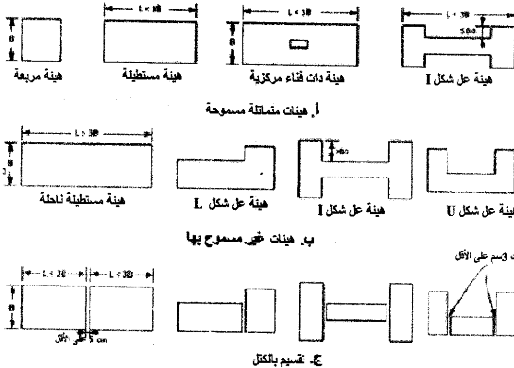
الشكل 30. هيئة في المسطح لبنانية بالطين
