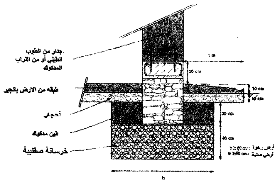
الشكل 49. أساس من خرسانة صقالية + مئترات من الخرسانة المسلحة + أعمدة الربط جدار - مئطرة
