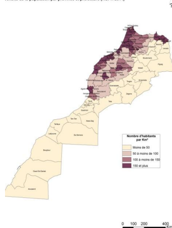
Densité de la population par province et préfecture (RGPH 2014)
