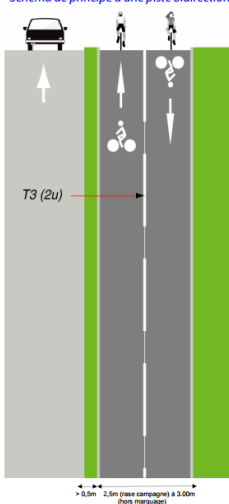
Schéma de principe d'une piste bidirectionnelle.
