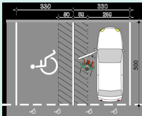
Stationnement perpendiculaire à la chaussée
