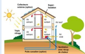
Schéma d'une maison passive
